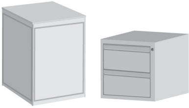
Νο 1 - Κύβος μεγάλων διαστάσεων M=0,55\text{ m} \times \text{Π}=0,55\text{ m} \times \text{Υ}=0,80\text{ m} Από αλουμίνιο και μελαμίνη Νο 2 - Συρταριέρα διαστάσεων M=0,43\text{ m} \times \text{Π}=0,48\text{ m} \times \text{Υ}=0,40\text{ m} Από γαλβανισμένο μέταλλο
